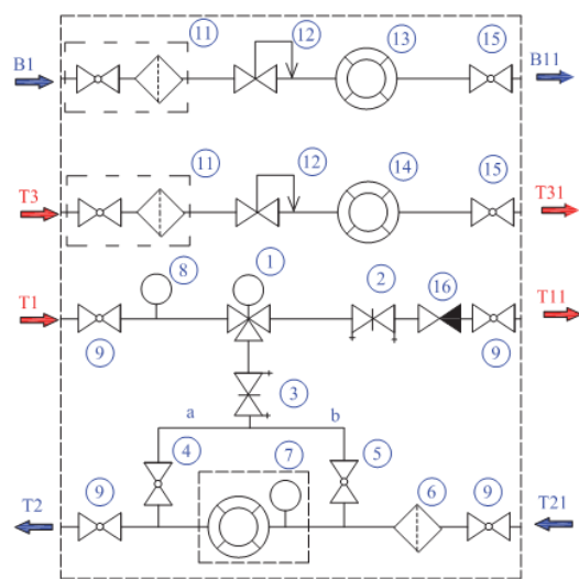
СОСТАВ СТАНЦИИ
